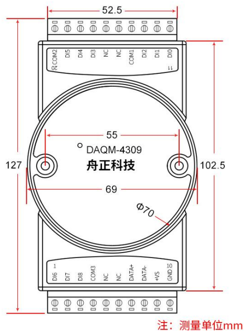
正视图
