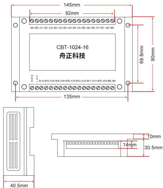
正、侧视图
