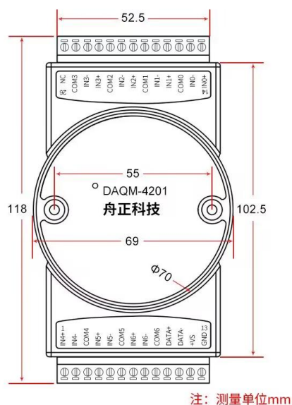
正视图
