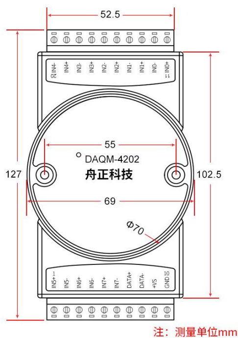
正视图
