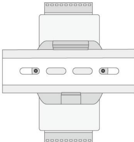
模块安装示意图
