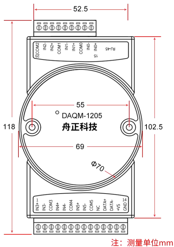
正视图
