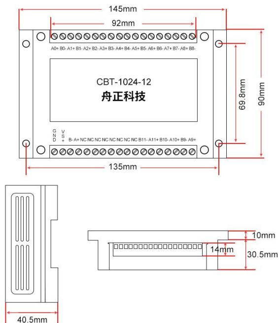
正、侧视图
