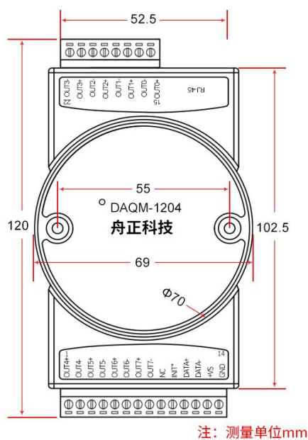
正视图
