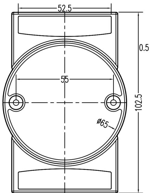
正视图
