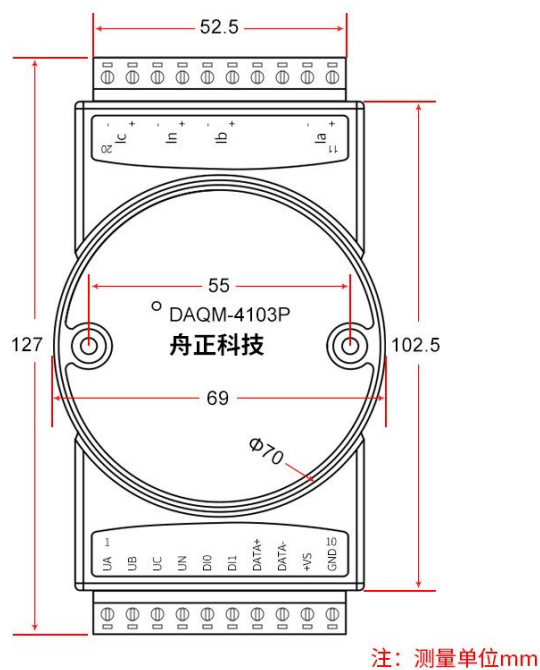
正视图
