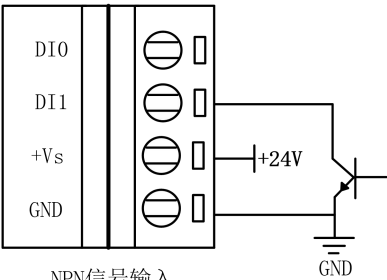
NPN信号输入
