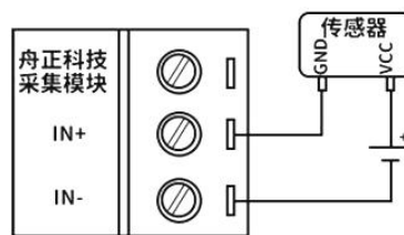
两线制传感器接法
