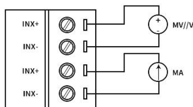
电压/电流可同时输入
