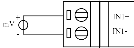
c) 电压信号接线方式
