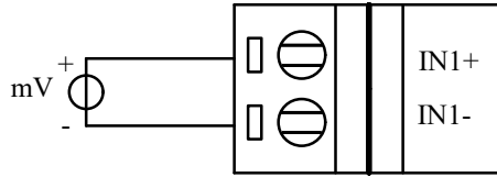
c) 电压信号接线方式 (以 IN1 通道为例, 其它通道类推)
