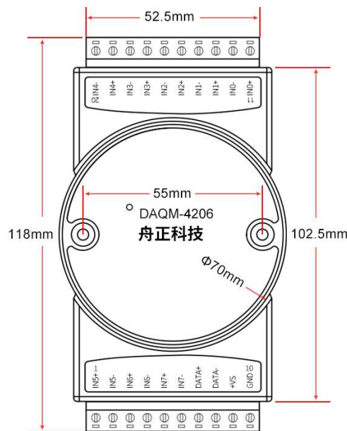
正视图
